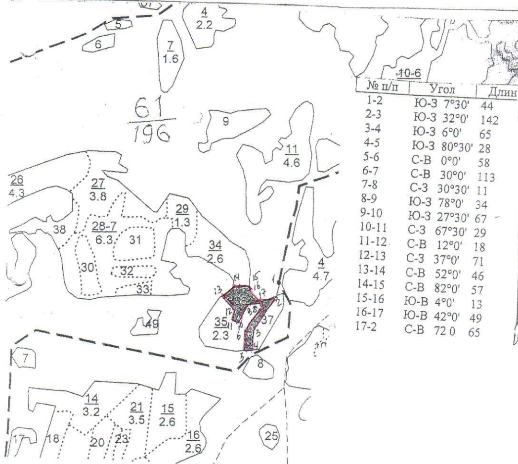
План участка, масштаб 1:10000
